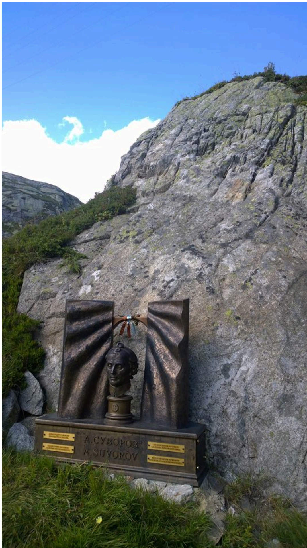
Суворову - победоносцу
