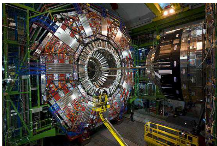
CMS - Компактный мюонный соленоид (© CERN)
